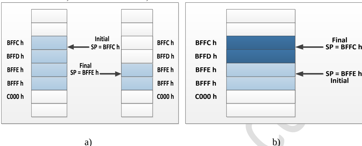
Figura 2. a)Extragerea din stivă; b)Depunerea în stivă.
